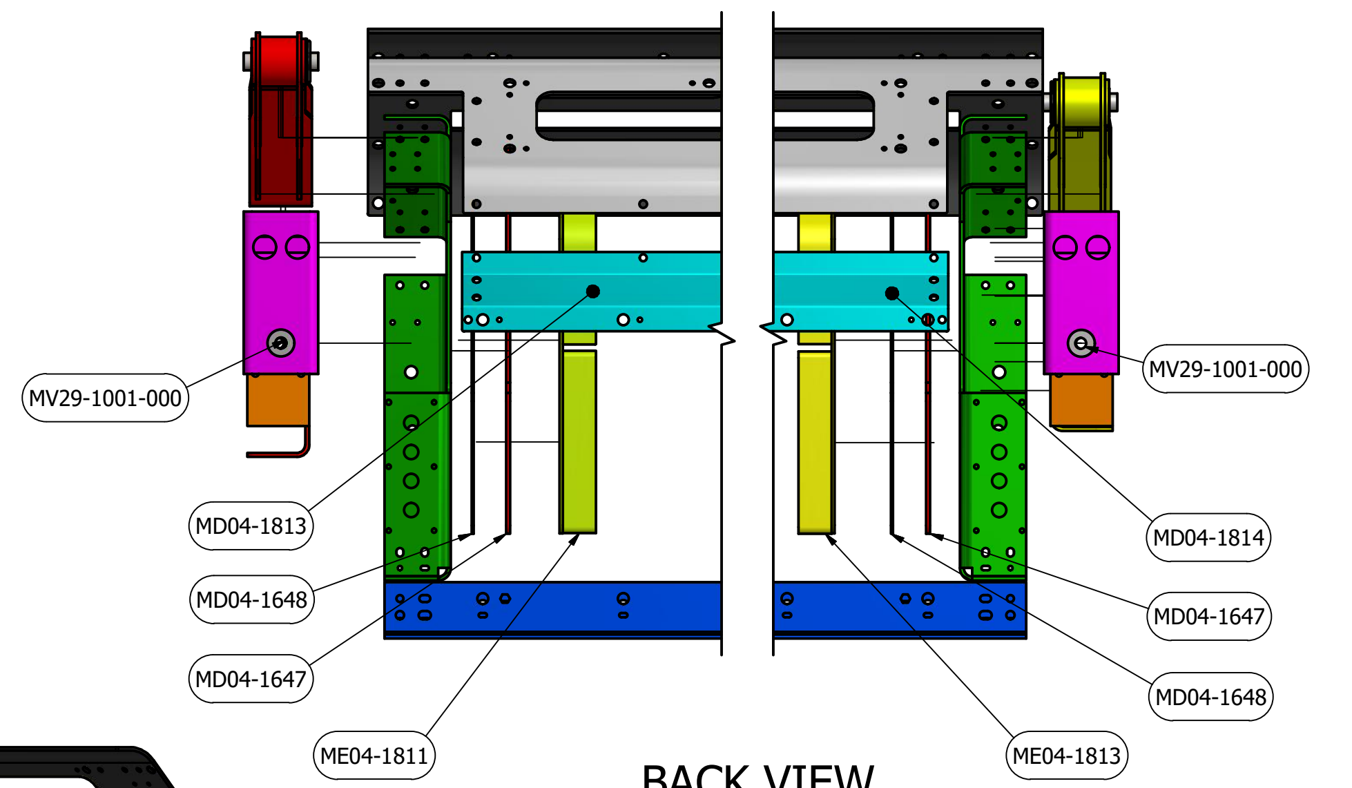
DETAIL B SCALE 0.16 : 1
